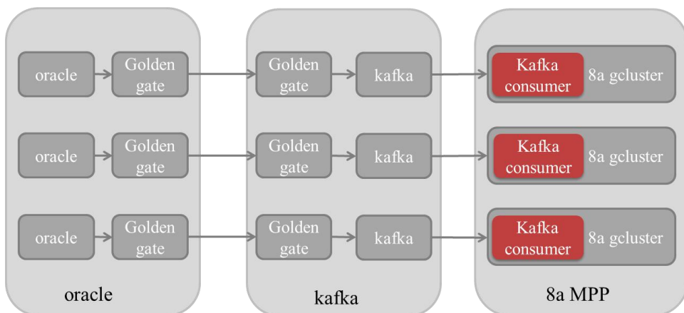
图 2-5 kafka 数据同步总体流程图
